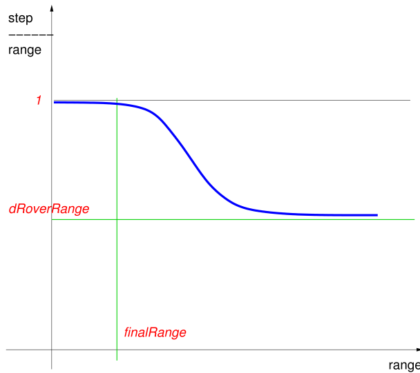
Fig. 8.1: Step limit.
